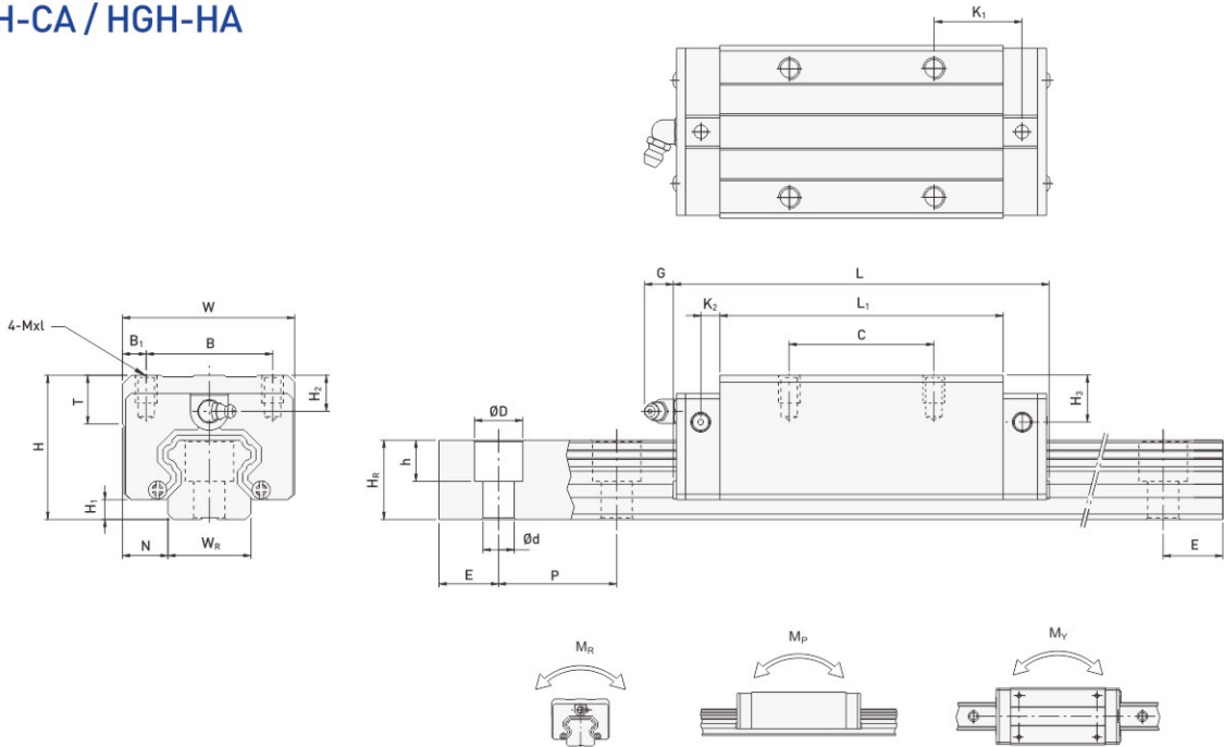
2-1-13 HG系列导轨尺寸表
