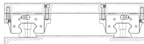
HGW型滑块装配螺栓取不同方向配置
