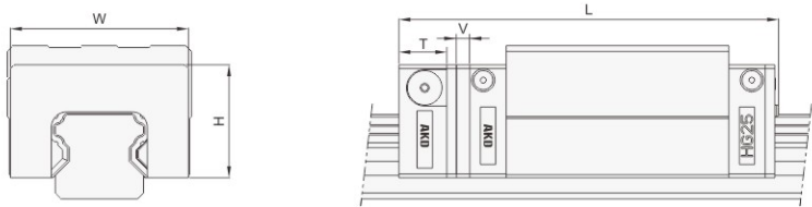
2-5-7 E2型式自润式直线导轨尺寸表
