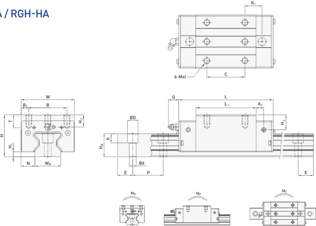
2-4-13 RG系列直线导轨尺寸表
