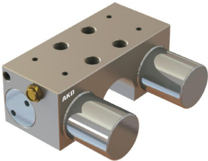
EZS-G系直线光轴用常闭钳制器
